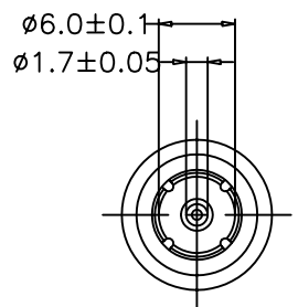
MINI RCA PLUG
