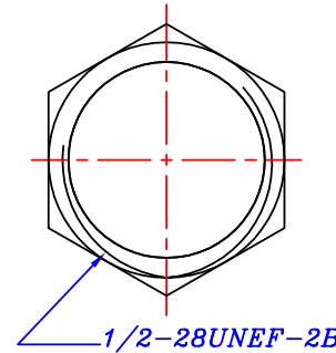
⑦ CLAMP NUT
